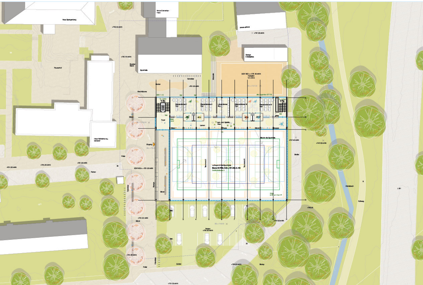
Grundriss Erdgeschoss 1:200
